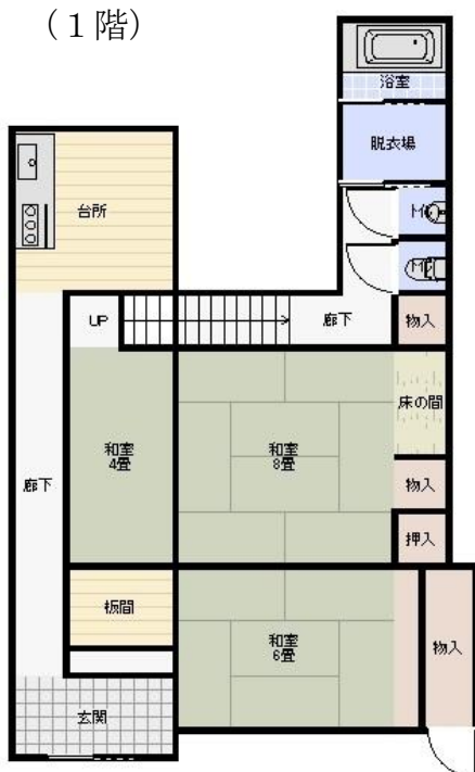
(間取り図)
